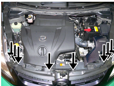
4: フロントグリル及びバンパーを固定している5ヶ所のクリップと2ヶ所のボルトを外します。
