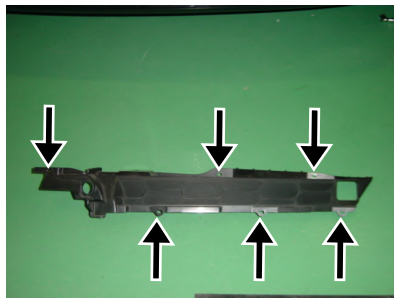
6: グリルブラケット 矢印部 6ヶ所のタッピングビスを外します。(下側の3ヶ所は短いドライバーを使用してください。)
