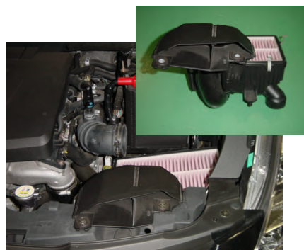
3: 純正エアクリーナーボックスをフレッシュエアダクトごと取り外します。純正エアクリーナーボックスからエアフロセンサーを取り外します。
