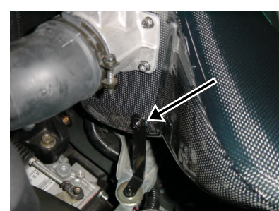
9: ラムエアインテークASSYを純正エアホースに差し込み車両に配置し、カーボンダクトケースをステアに仮組みします。(ビスA使用)
