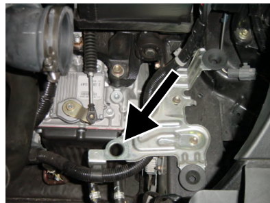
1: 矢印部のインシュレーションラバーを外します。
