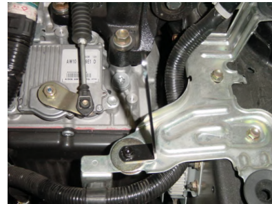
2: エアクリーナーブラケットの上下にワッシャーを挟み、その上にステアを仮組みします。(ビスB、ナット使用)
