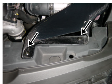
10: カーボンダクトケースを丸ビスで2ヶ所固定します。
