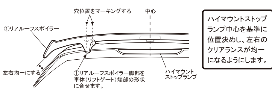
図2 ①リアーフスポイラーの取付け位置
