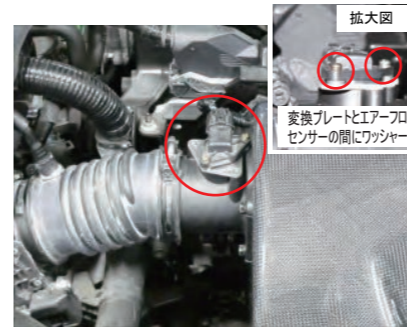
16. ビスFとワッシャーを使用してエアフローセンサーを取付けます。
