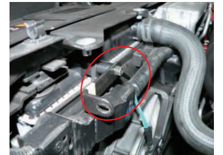
12. スパーサーを挟みビスDでステーBを取付けます。
