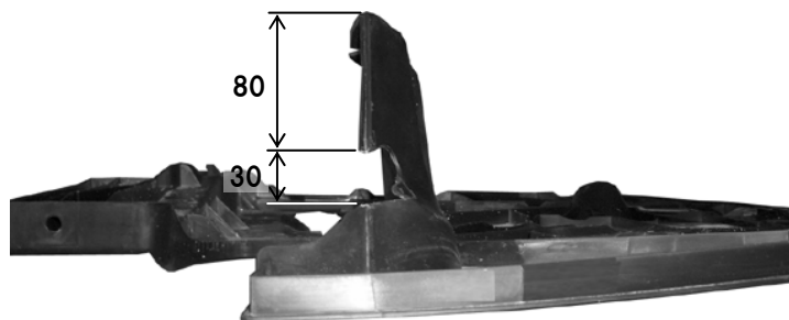
車両後方より見た図
