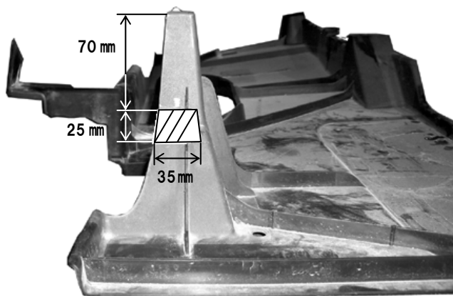
車両後方より見た図
