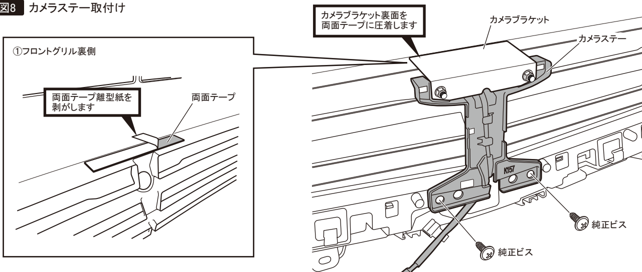
図9 フロントバンパー復元
