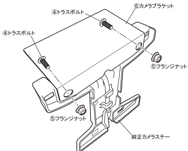
図7 カメラブラケット取付け
