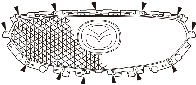
図6 ロアグリルモールディング、ロケーターピンブラケット、アッパーフェースの復元
