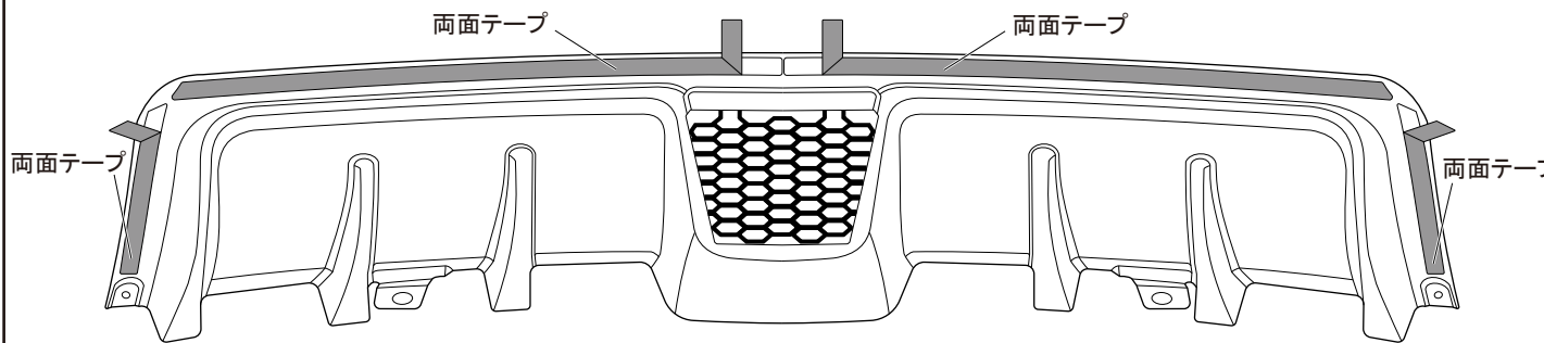
図5 ①リアアンダーガーニッシュ取付け
