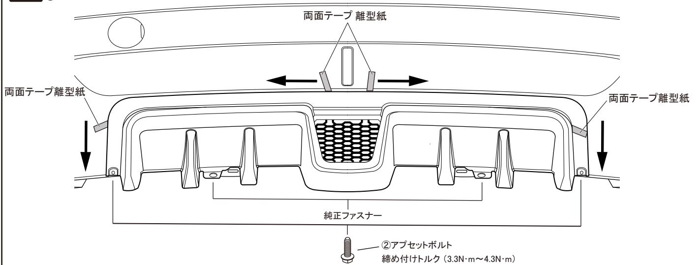
図5 ①リアアンダーガーニッシュ取付け
