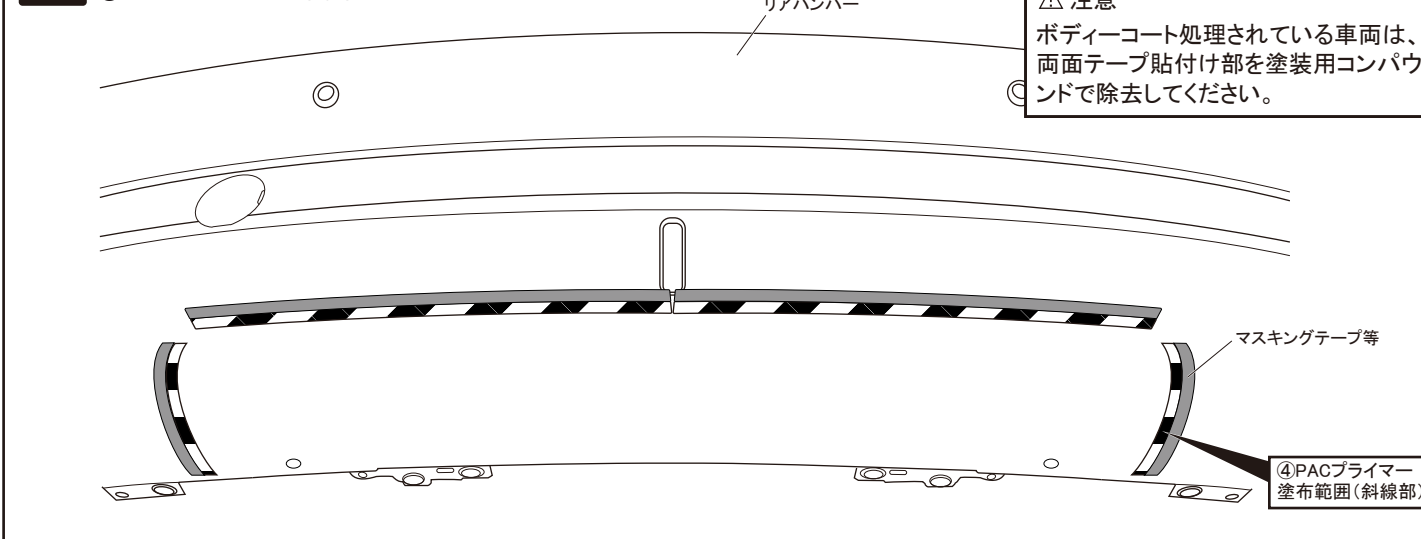
図4 ①リアアンダーガーニッシュ裏面
