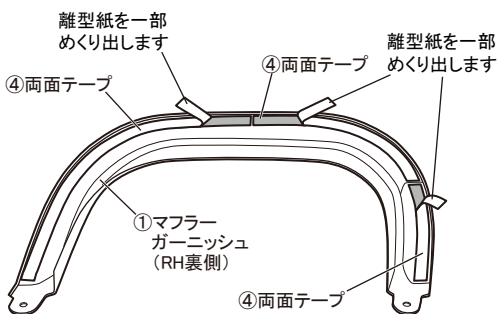
図3 両面テープ貼付け位置
