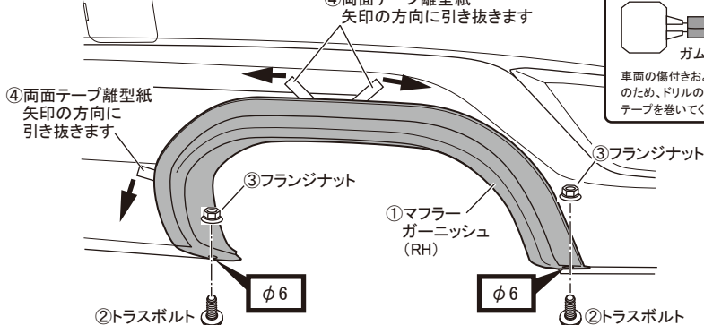
図4 ①マフラーガーニッシュ取付け ※図は右側です。左右同作業
