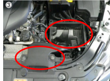
③ フレッシュエアダクトとエアークリーナーケースを取外します。
