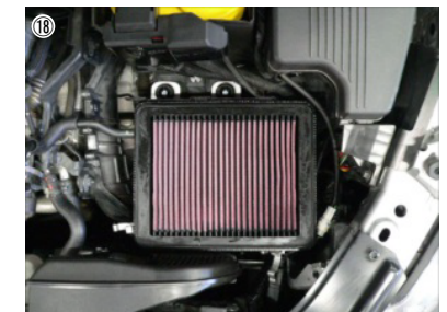
⑱ エアークリーナーケースからマウンティングラバー2個とクリップ2個を取外します。
