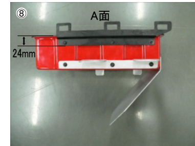
⑧ ブラケットAとアルミステーAを取付けます。(ブラケットA、Bの基本取付位置は上図を参照)
