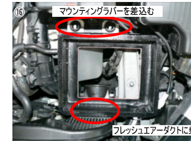
⑯ エアークリーナーカバー奥側の爪をブラケットAの穴に挿入してカバー閉め、クリップ2か所を固定します。
