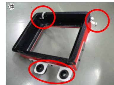
⑬ エアークリーナーケースから外したクリップとマウンティングラバーをステーに移設します。
