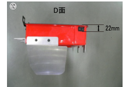
⑫ ブラケットB、ヒートプレートを取付けます。(ブラケットA、Bの基本取付位置は上図を参照)
