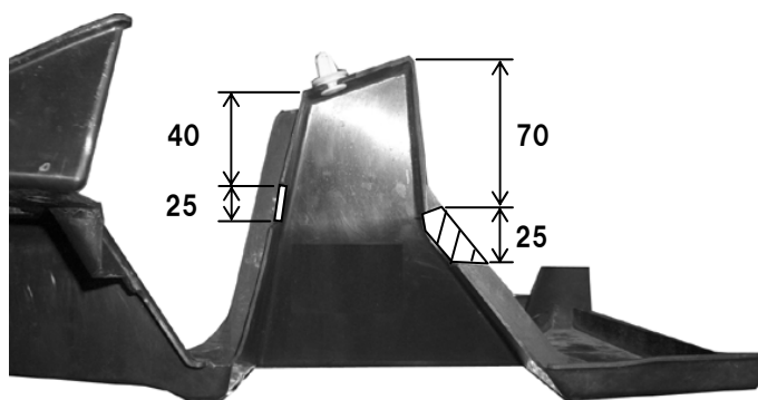
側面図
