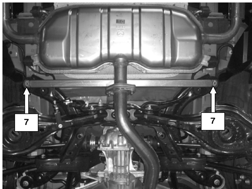
取付方向
