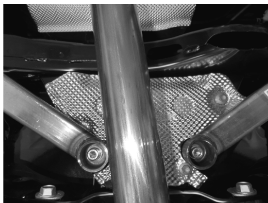
取付図
