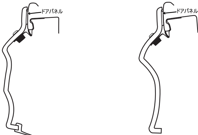
フロントバイザー 取付け断面図
