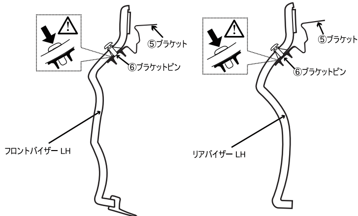
フロントバイザー 断面図
