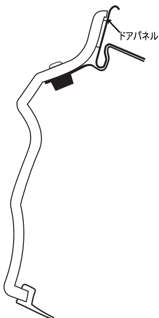
②フロントバイザー取付け断面図
