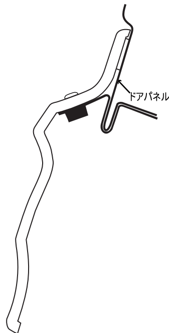
④リアバイザー取付け断面図
