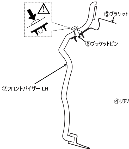
②フロントバイザー断面図
