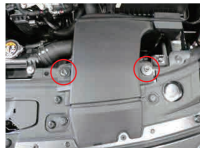
3. フレッシュエアダクトを固定しているボルトを取外します。
