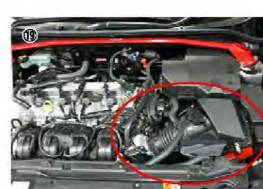
⑲ クリーナーケース上側のエアホース部分をスロットルに差し込み、フィルターカバーに取り付けます。
