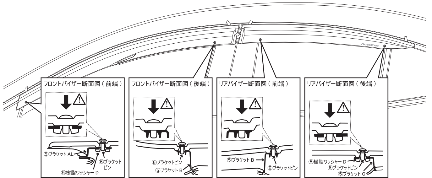
ブラケットと樹脂ワッシャーの固定方法(フロントパイザー)
