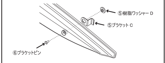
ブラケットと樹脂ワッシャーの固定方法(リアパイザー)
