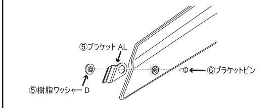
ブラケットと樹脂ワッシャーの固定方法(フロントパイザー)
